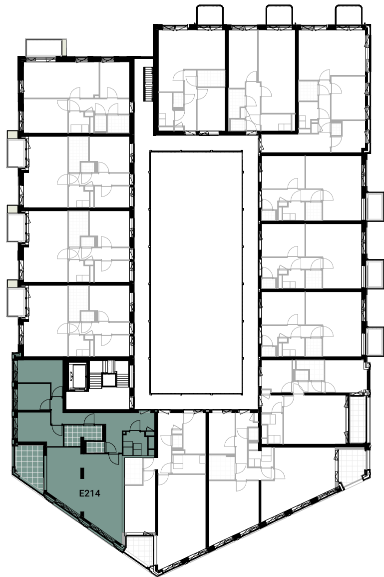
2e verdieping
